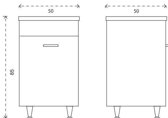
140-101-5050 1 anta
