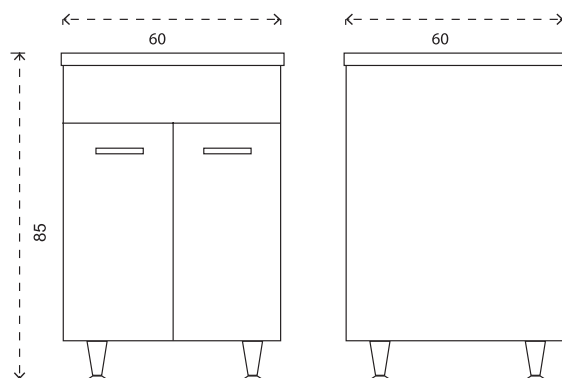
140-101-6060 2 ante
