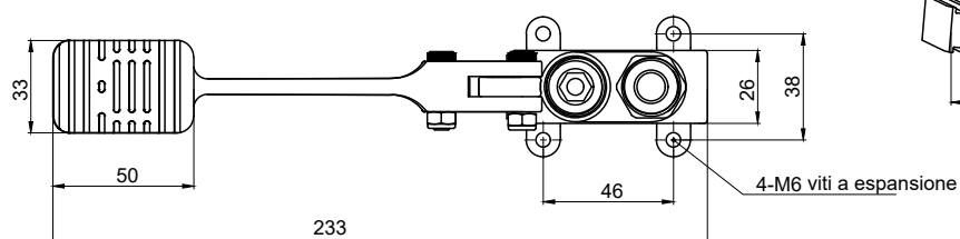
installazione orizzontale
