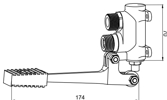
installazione verticale
