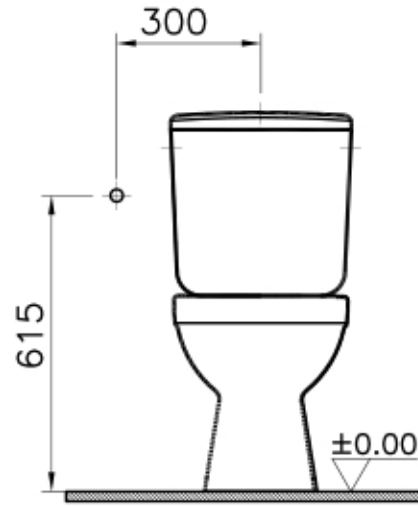
Yandan girisli Side inlet Zulauf seitlich
