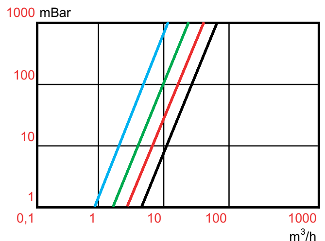
Diagramma log. perdite di carico / portata Load losses / flow rate log.graph
